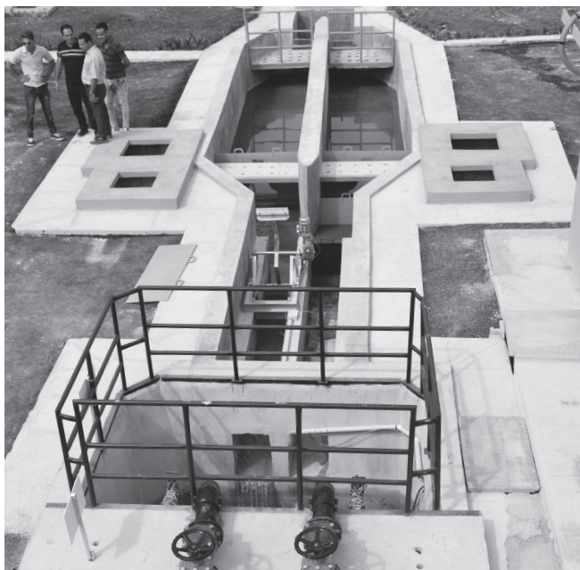
Canal Desarenador Vista Superior
